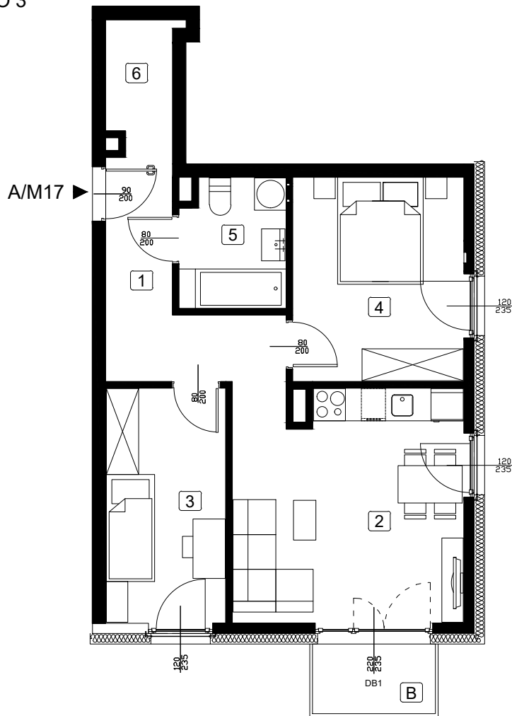
RZUT KONDYGNACJI 3 PIĘTRA
