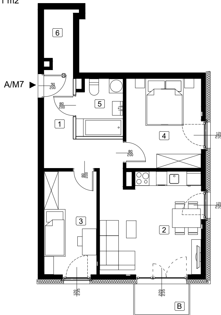
RZUT KONDYGNACJI 1 PIĘTRA
